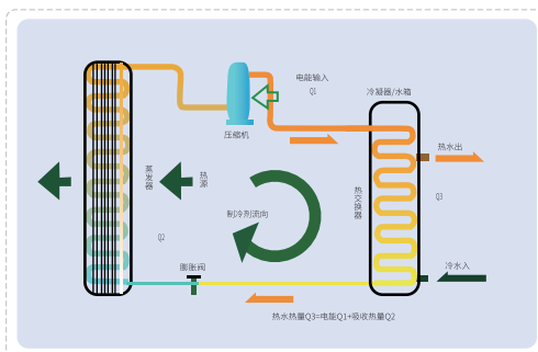
热泵热水机组工作原理
