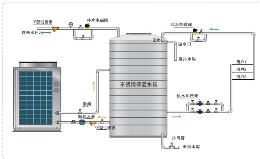
商用热泵热水机组安装图
